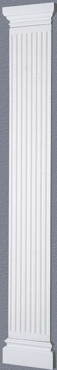
PILASTRA Nº 4 Altura total: 138 cms. Pieza Central Ref.: 1112 Dim.: 118 x 17,4 cms. Base Inferior Ref.: 1113 Dim.: 10,1 x 20,8 cms. Base Superior Ref.: 1114 Dim.: 7,9 x 21,2 cms.
