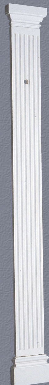
PILASTRA N° 3 Altura total: 138 cms. Pieza Central Ref.: 1109 Dim.: 120 x 11,7 cms. Base Inferior Ref.: 1110 Dim.: 10,1 x 15,3 cms. Base Superior Ref.: 1111 Dim.: 7,6 x 15,7 cms.
